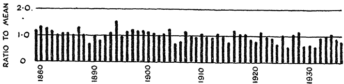
ओरेगन, डेलीज पर कोलम्बिया नदी। (औसत, ११.४४ इंच। समय १८७६-१९३६)
